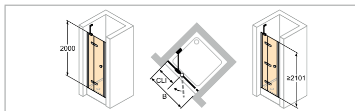
Linksbefestigung
